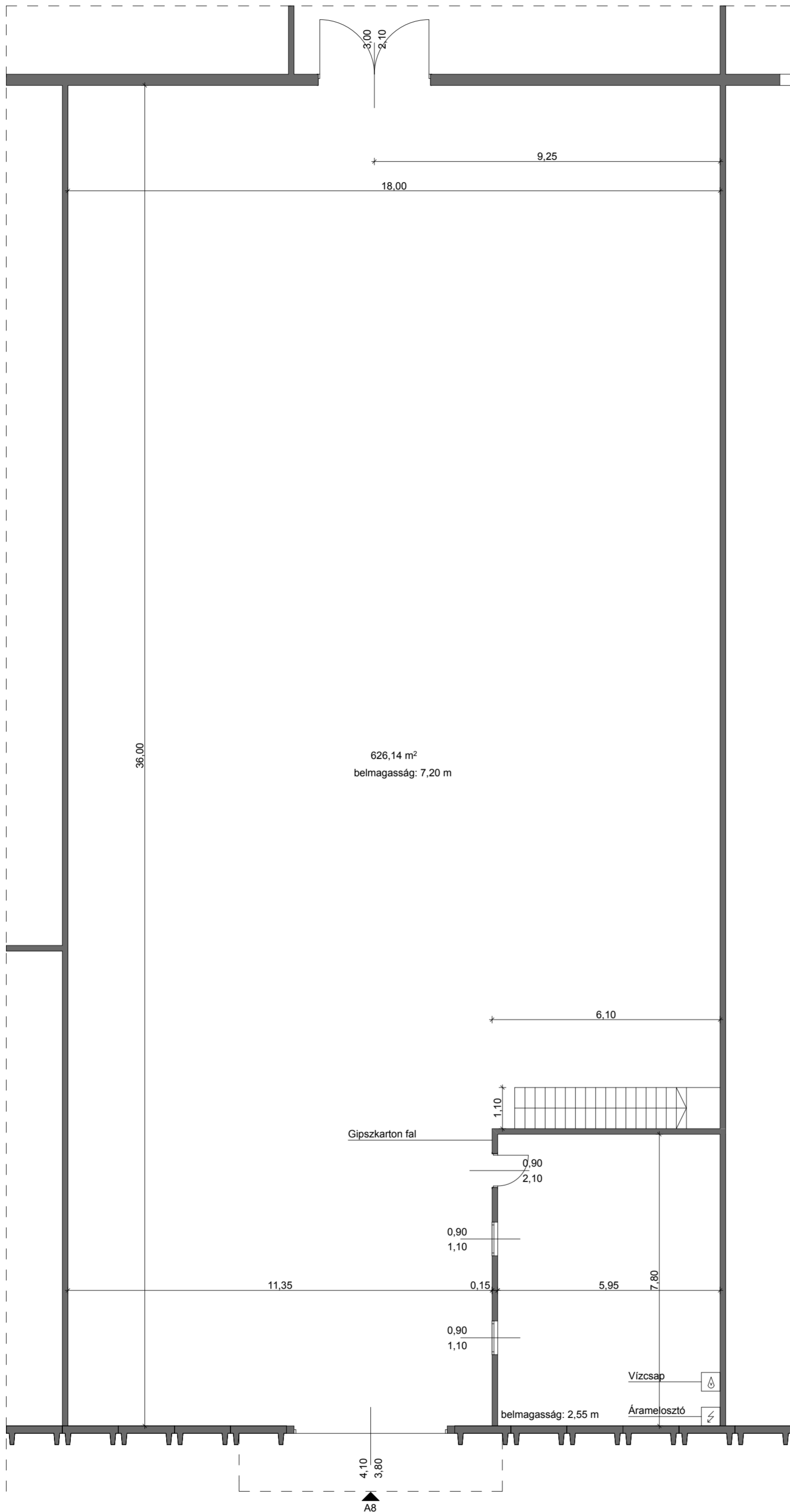
Földszinti alaprajz
